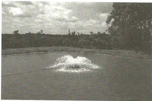
Aerador em funcionamento.
